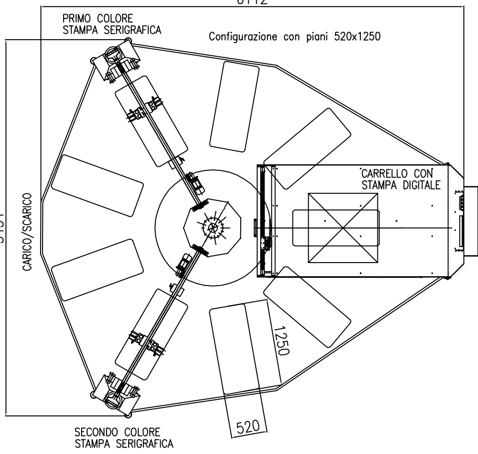
ALFA PLUS 2/9 CON CARRELLO PER STAMPA DIGITALE SD 100
