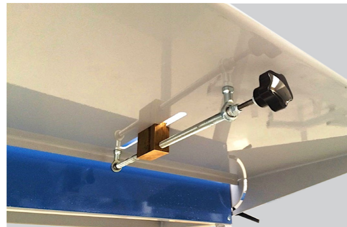
REGOLAZIONE ANGOLO DI AFFILATURA SHARPENING ANGLE ADJUSTMENT
